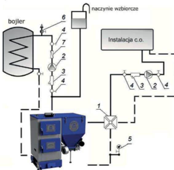
Rys. 3. Przykładowy schemat podłączenia kotła do instalacji grzewczej (centralnego ogrzewania) z wykorzystaniem zaworu mieszającego – czterdrogowego, gdzie: 1 – zawór czterdrogowy, 2 – pompa c.o., 3 – filtr siatkowy, 4 – zawór odcinający, 5 – manometr z zaworem, 6 – odpowietrznik automatyczny, 7 – zawór zwrotny
