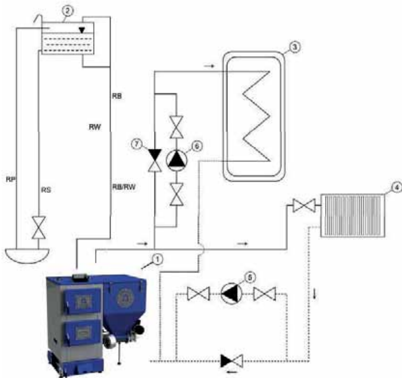
Rys. 4. Schemat poglądowy zabezpieczenia kotła DWOREK ZPS EKO BLUE w układzie grzewczym otwartym, gdzie: 1 – kocioł, 2 – naczynie wzbiornicze (przelewowe), 3 – zasobnik c.w.u., 4 – obieg grzewczy, 5 – pompa c.o. (obiegowa), 6 – pompa c.w.u. (obiegowa), 7 – zawór różnicowy, RO – rura odpowietrzająca, RS – rura sygnalizacyjna, RB – rura bezpieczeństwa, RW – rura wzbiornicza, RP – rura przelewowa
