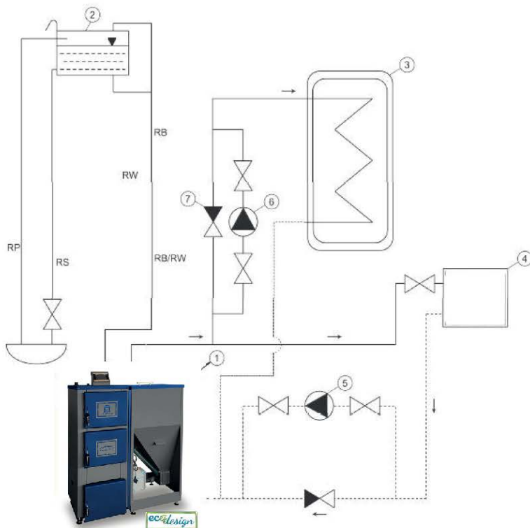
Rys. 4. Schemat poglądowy zabezpieczenia kotła DWOREK BIO COMFORT BLUE 10-50kW w układzie grzewczym otwartym, gdzie: 1 – kocioł, 2 – naczynie wzbiórcze (przelewowe), 3 – zasobnik c.w.u., 4 – obieg grzewczy, 5 – pompa c.o. (obiegowa), 6 – pompa c.w.u. (obiegowa), 7 – zawór różnicowy, RO – rura odpowietrzająca, RS – rura sygnalizacyjna, RB – rura bezpieczeństwa, RW – rura wzbiórcza, RP – rura przelewowa
