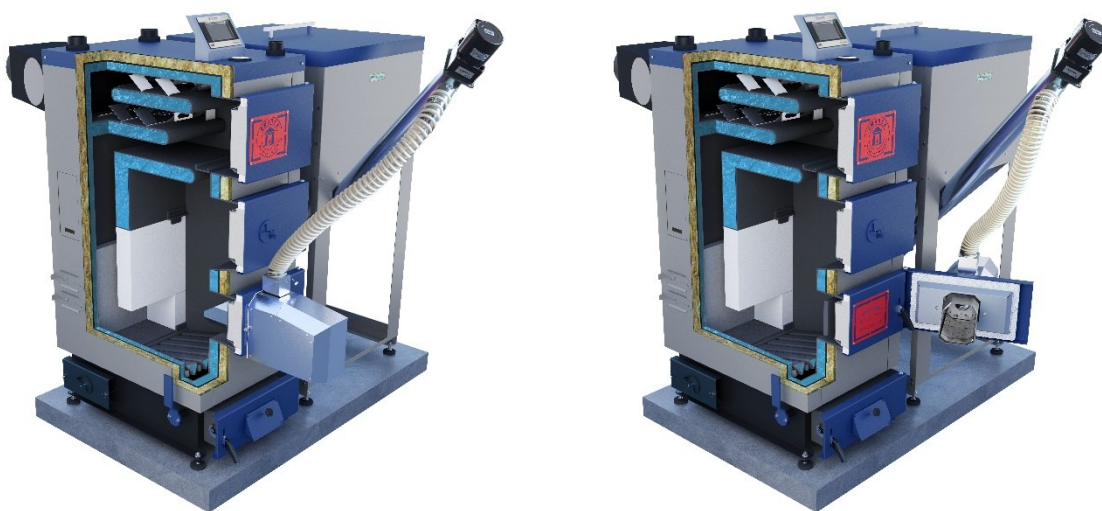
Rysunek 1. Widok i przekrój kotła c.o. MZN EKO PLUS DUO
